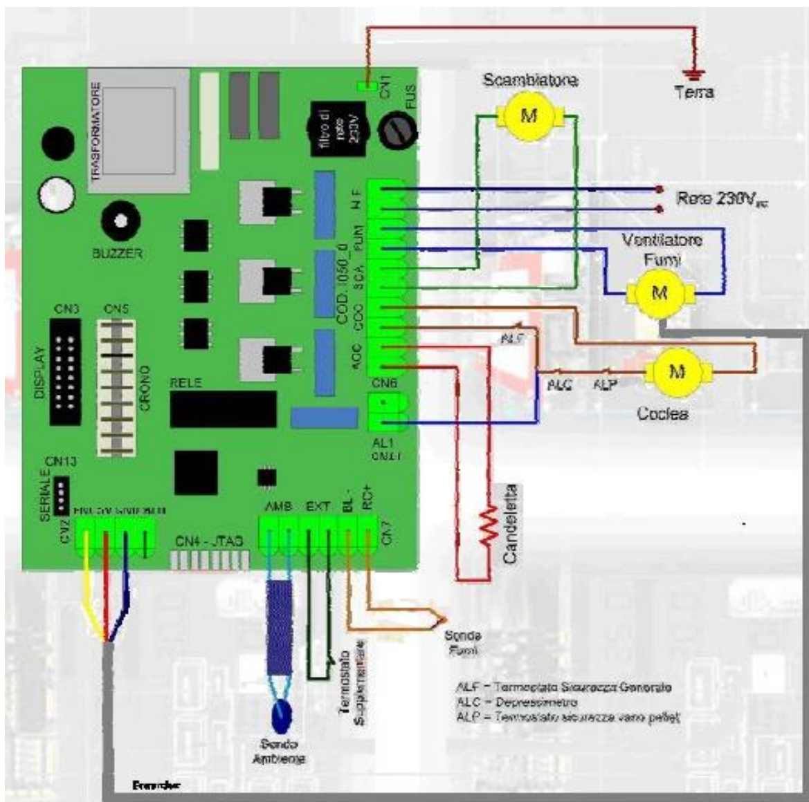
Slika 32. Elektronska kartica
